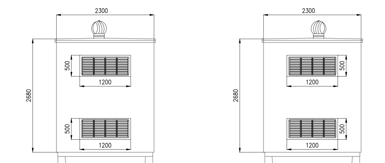
Dettagli cabina di trasformazione - Scala 1:50
