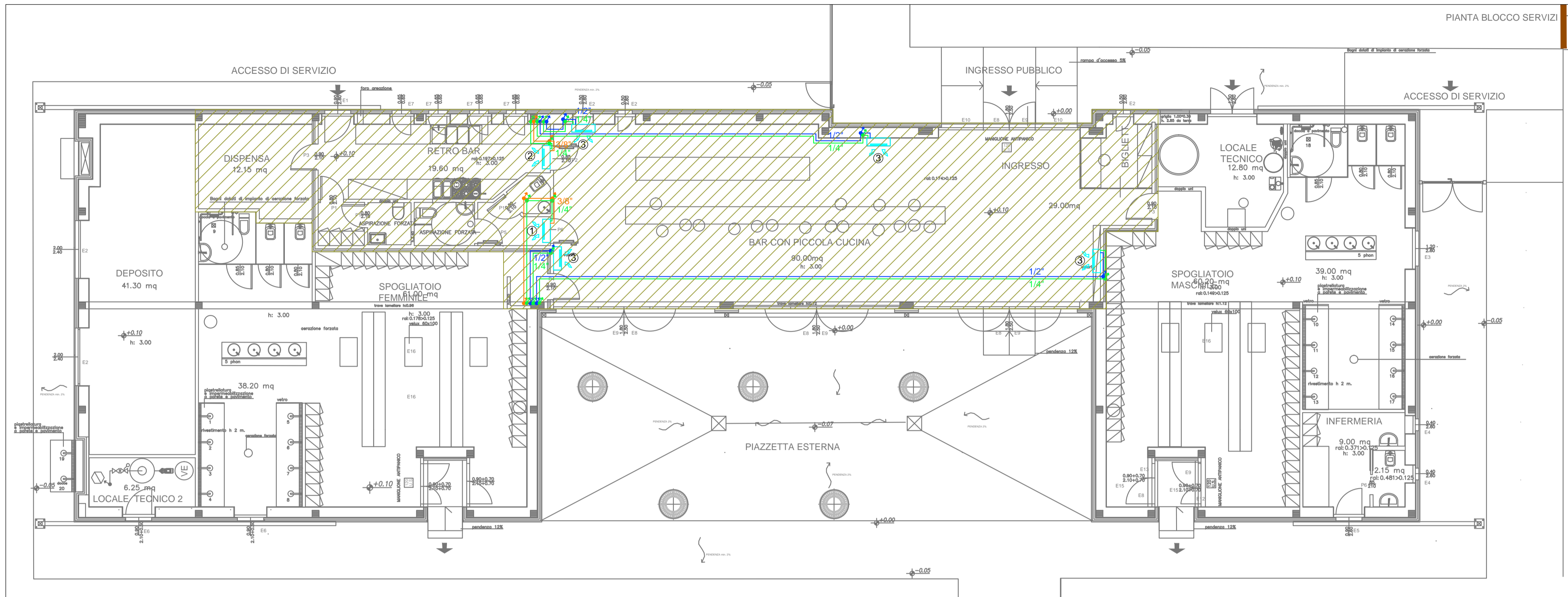
PIANTA PIANO TERRA IMPIANTO CLIMATIZZAZIONE BAR E SPOGLIATOI - scala 1:100
