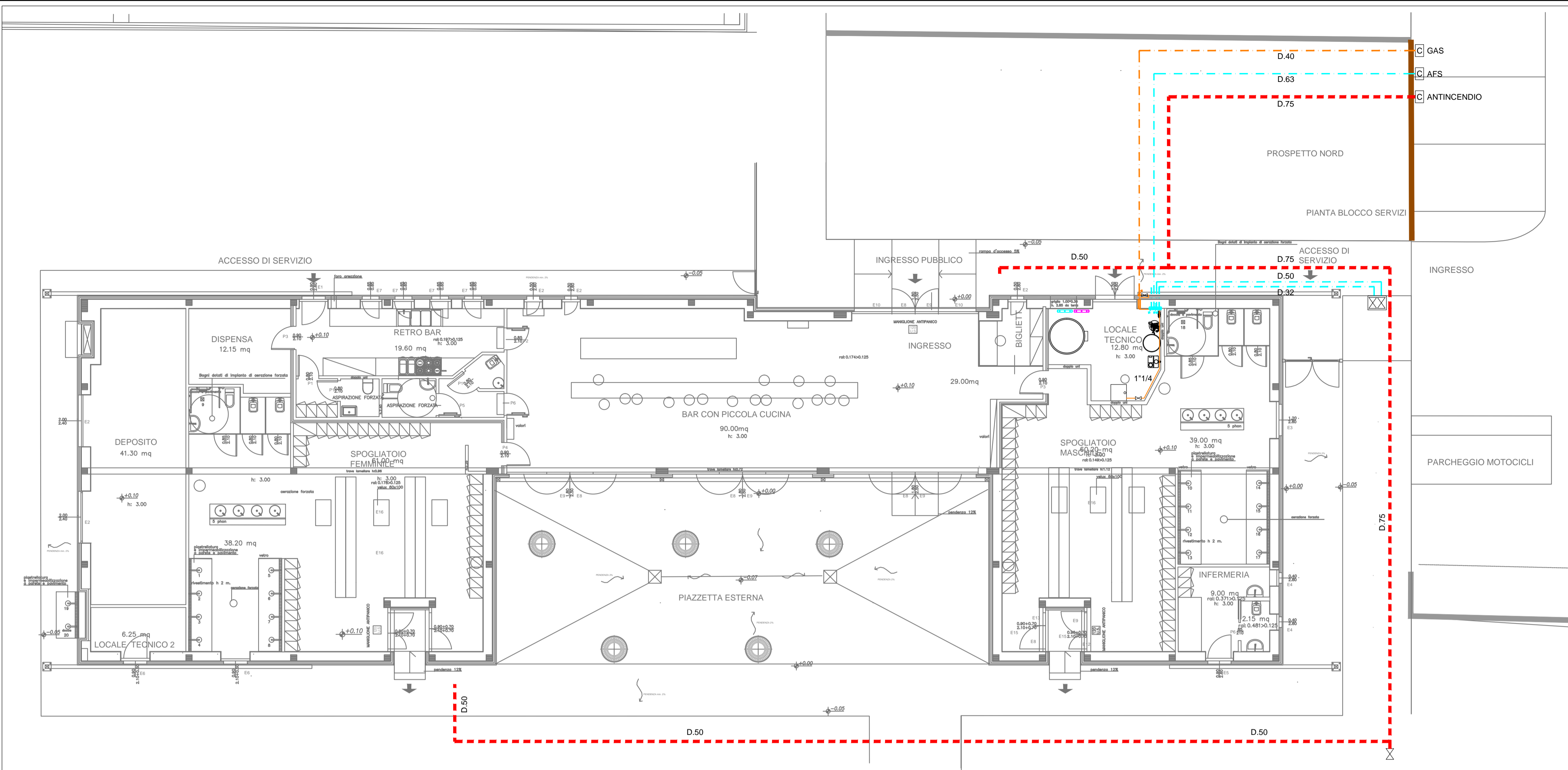
PLANIMETRIA IMPIANTI RETI ESTERNE BAR E SPOGLIATOI - scala 1:100
