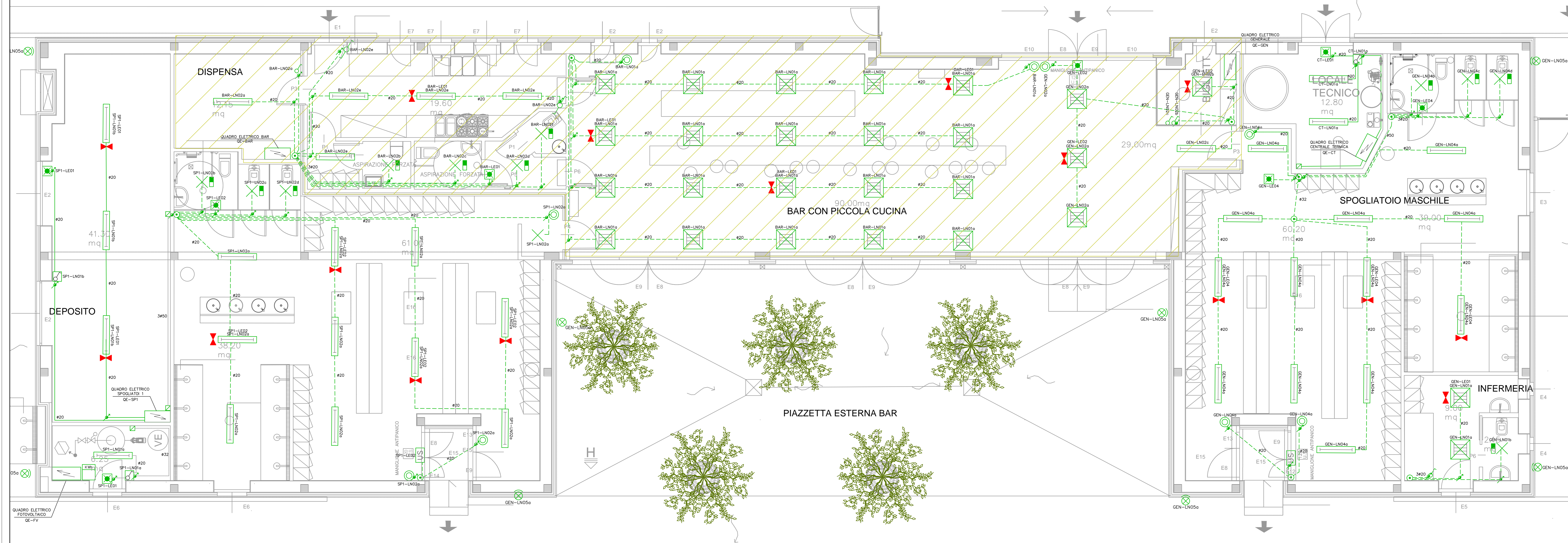
PLANIMETRIA IMPIANTO DI ILLUMINAZIONE BAR E SPOGLIATOI - scala 1:50
