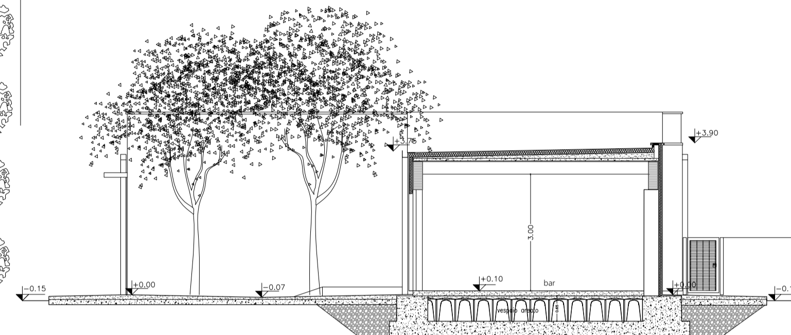
SEZIONE F-F
