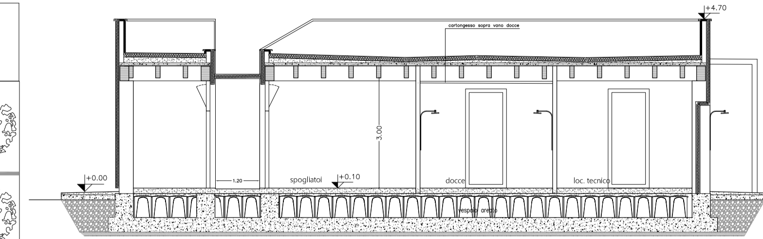
SEZIONE E-E
